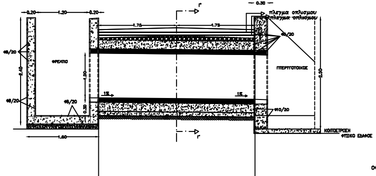
ΤΟΜΗ Γ - Γ'
