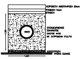
ΤΟΜΗ Γ - Γ'
